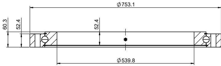
VIEW A-A
