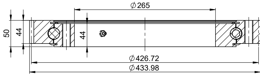
VIEW A-A
